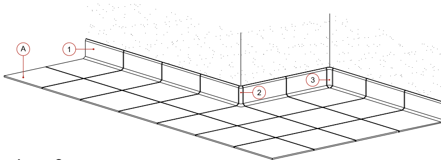
art. zoccolo ad appoggio cm 10x20 - 4"x7 7/8 "
