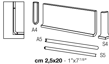
Zoccolo a raccordo a taglio retto Cove base - straight top Plinthe à gorge avec bord vif Hohlkehlssockel (scharfkantig)
