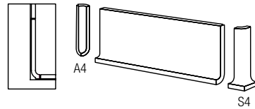
Zoccolo a raccordo a taglio retto*
