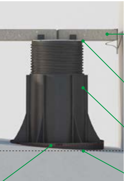
Pavimentazione Paving tile Revêtement de sol Fußbodenbelag Testa NM NM head Tête NM Kopf NM Supporto regolabile “NEW-MAXI” “NEW-MAXI” adjustable paver support Support réglable “NEW-MAXI” Verstellbare Stütze “NEW-MAXI” Pendenze fino al 5% Gradient up to 5% Pentes jusqu'à 5% Neigungen bis zu 5%
