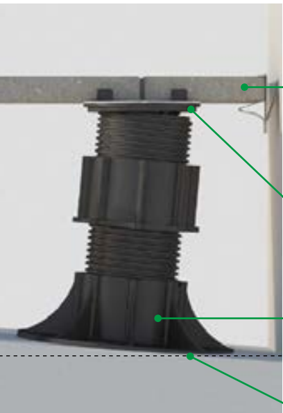
Pavimentazione Paving tile Revêtement de sol Fußbodenbelag Testa autolivellante Self-levelling head Tête auto-nivelante Selbstnivellierender Kopf Supporto regolabile “ETERNO” Adjustable paving support “ETERNO” Support réglable “ETERNO” Verstellbare Stütze “ETERNO” Pendenze fino al 5% Gradient up to 5% Pentes jusqu'à 5% Neigungen bis zu 5%
