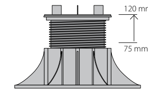
Supporto a testa autolivellante
