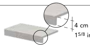
16,5x30 . 6 1 / 2 "x12" ELEMENTO A L MONOLITICO G3NS15ELM HNS 15
