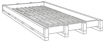
CASSA 137×292×42 cm CRATE 54"x115"x16" PESO VUOTO empty weight 149 kg
