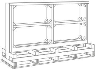
RACK PALLET 75×290×160 cm 30"x114"x63" PESO VUOTO empty weight 150 kg
