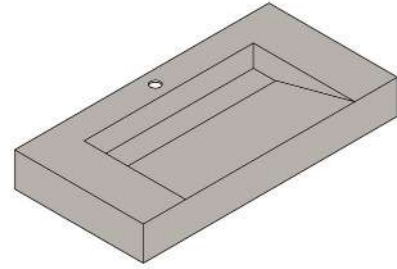
S/P Lavabo integrado 90 seno rampa C Dim. 455P x 900L x 120H mm | CC945
