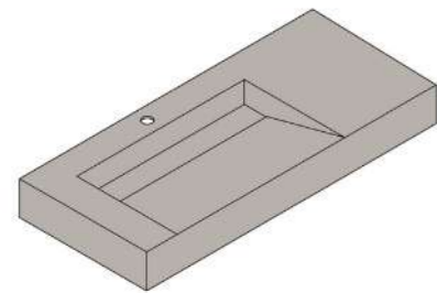
S/P Lavabo integrado 119 seno rampa L-I Dim. 455P x 1190L x 120H mm | CC950
