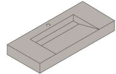
S/P Lavabo integrado 119 seno rampa C Dim. 455P x 1190L x 120H mm | CC950
