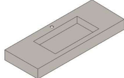
S/P Lavabo integrado 119 seno recto C Dim. 455P x 1190L x 120H mm | CC950
