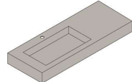
S/P Lavabo integrado 119 seno recto L-I Dim. 455P x 1190L x 120H mm | CC950
