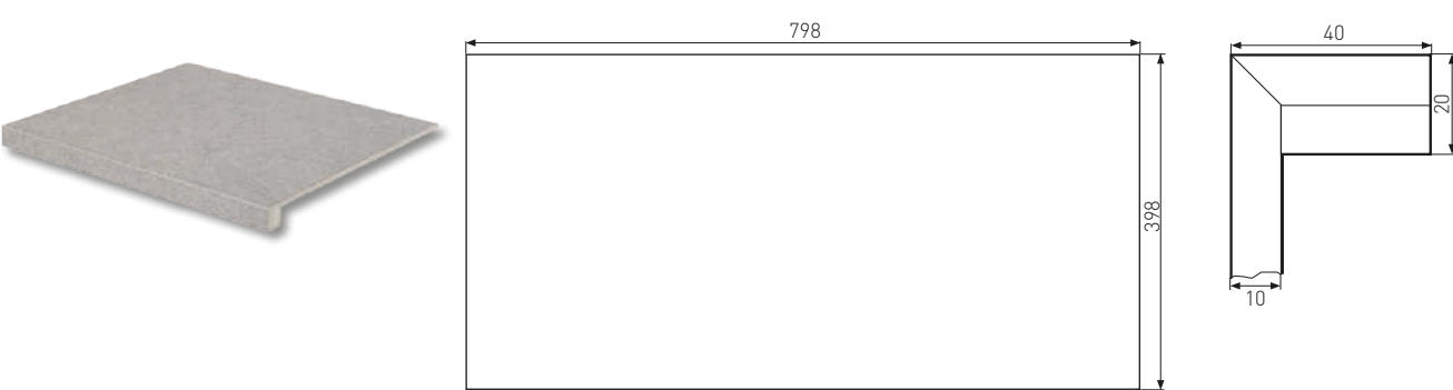
Stufenformteil | special step tile | DCF84... | 398×798×10 mm
