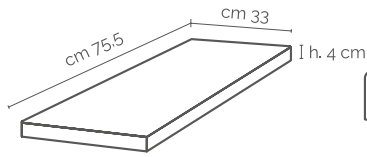
Angolare Assemblato 75.5x33cm
